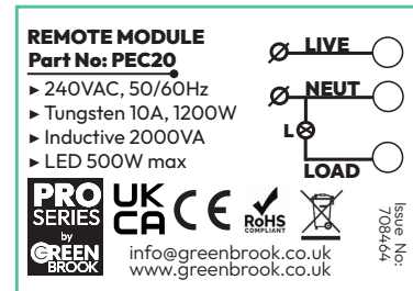
PEC20 Wiring Label
